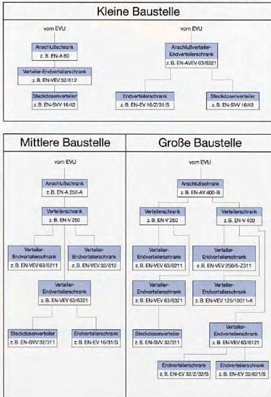
Anschluß verschiedener Baustromverteiler untereinander – Beispiele
